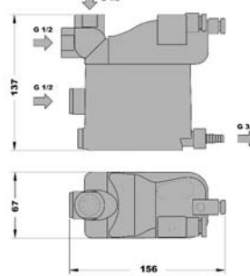
ED3030 1,1 kg
