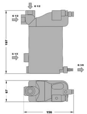
ED3100 1,5 kg
