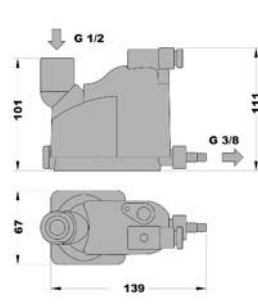
ED3004 0,6 kg
